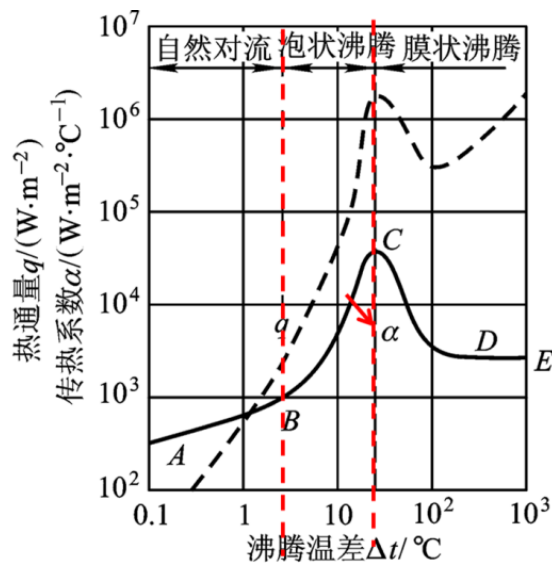
大容积饱和沸腾曲线
