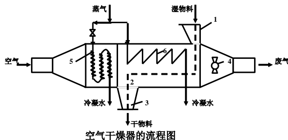
1—进料口；2—干燥室；3—卸料口；4—抽风机；5、6—空气加热器
