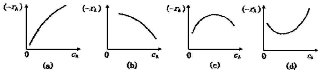
图7-2 反应速率与浓度的几种关系
