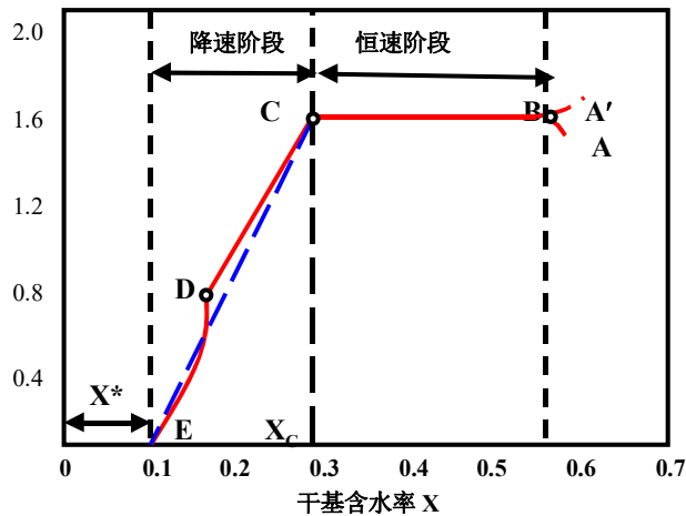
恒定干燥条件下的干燥速率曲线
