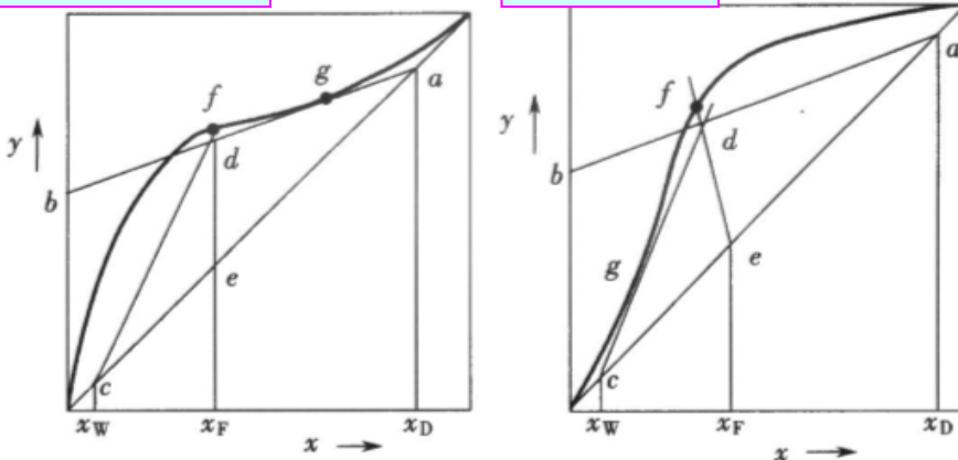
(a) (b) 不正常平衡曲线的 R_{\min} 的确定
