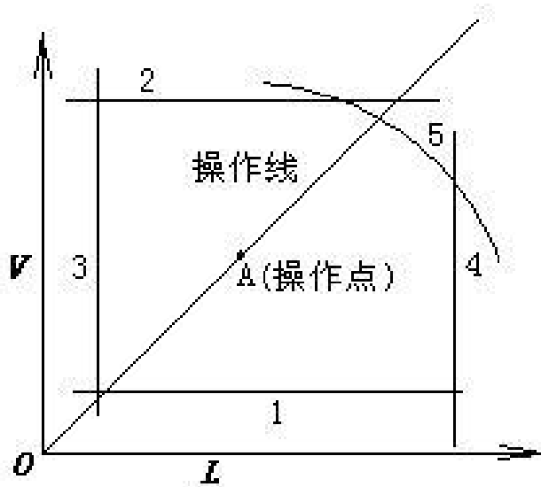
塔板的负荷性能图
